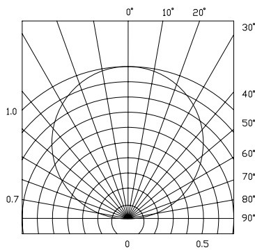
发光角度图解
