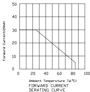
正向电流递减曲线图
